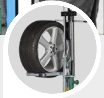
Kapacitet 60 kg. (Udvendig hjuldiameter max. 820 mm.)
